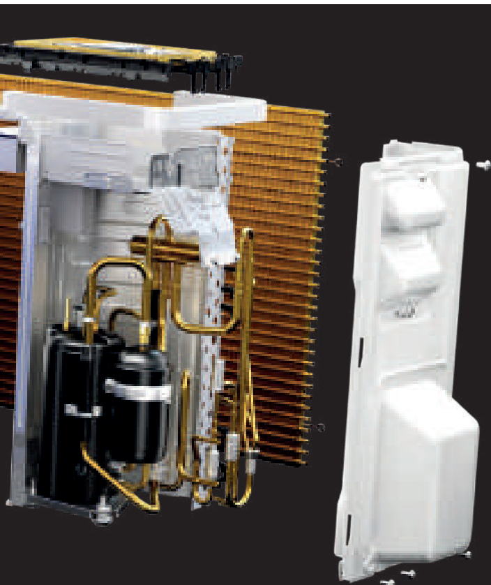
Standardowy kanał powietrza
